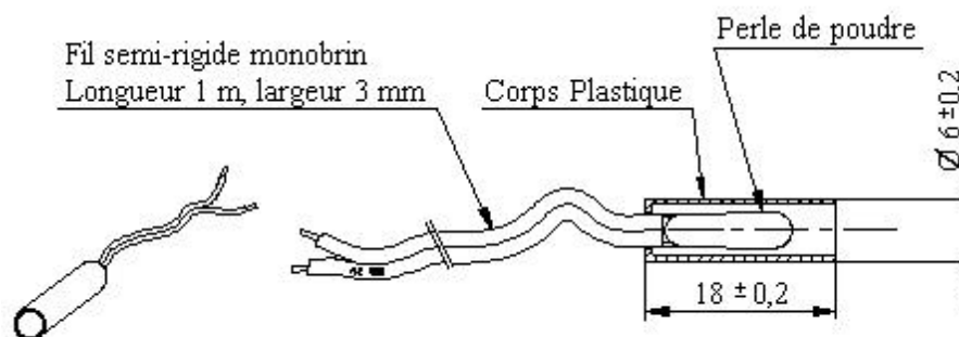
Inflammeur DAVEY-BICKFORD
