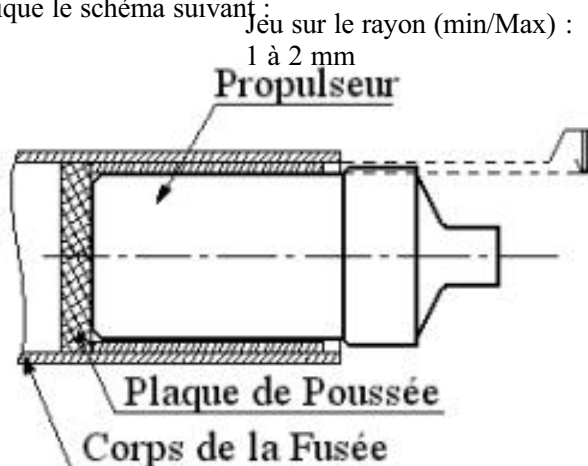
Montage avec moteur CARIACOU
